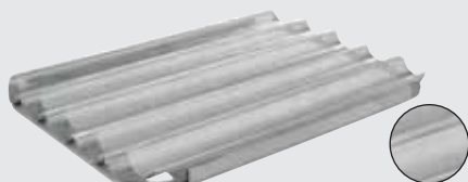
δίσκος αλουμινίου διάτρητος για 5 μπαγκέτες 20444994 60x40 cm
